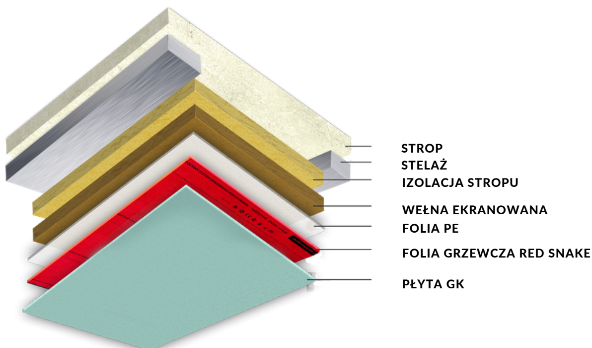
SCHEMAT UŁOŻENIA NA SUFICIE
