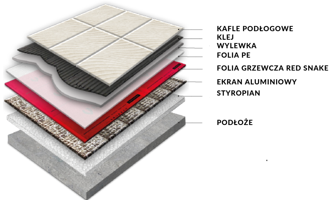
SCHEMAT UŁOŻENIA NA PODŁODZE Z PŁYTKAMI
